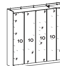
Para um bom funcionamento das portas é necessário o chão estar bem nivelado e os fundos no esquadro.
