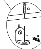
Para um bom funcionamento das portas é necessário o chão estar bem nivelado e os fundos no esquadro.
